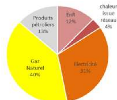
Répartition (852 GWh/an) des consommations dans l'habitat par source d'énergie en 2016 (source : BASEMIS, Air Pays de La Loire)
